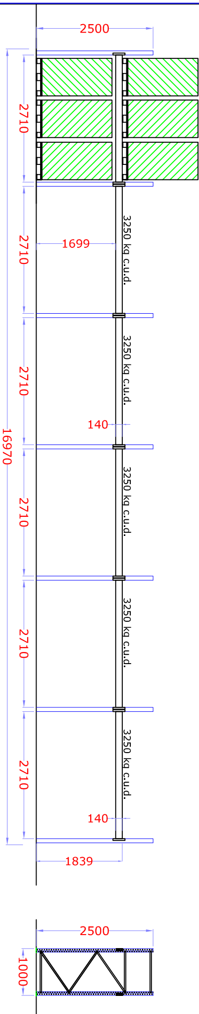
Prospetto frontale
