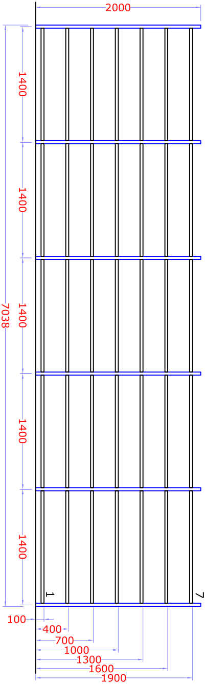
Prospetto frontale
