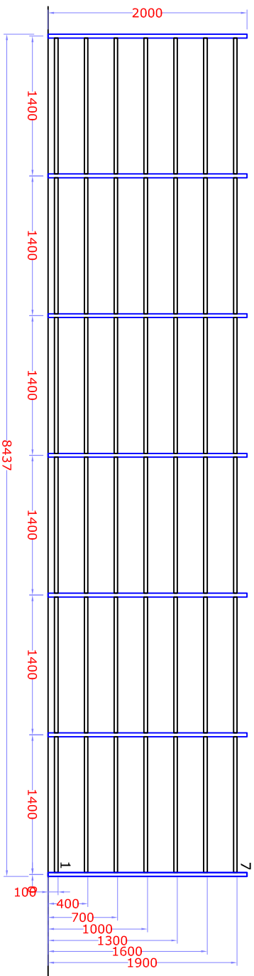
Prospetto frontale
